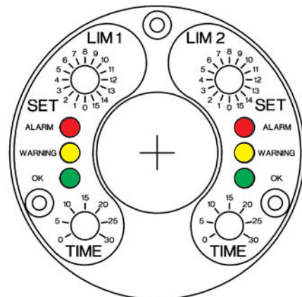
Abb. 10 Bedienelemente
