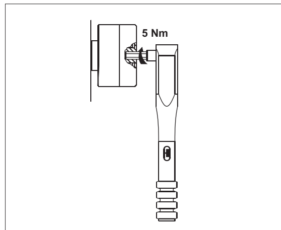
Abb. 13: Gehäusedeckel mit Drehmomentschlüssel anziehen
