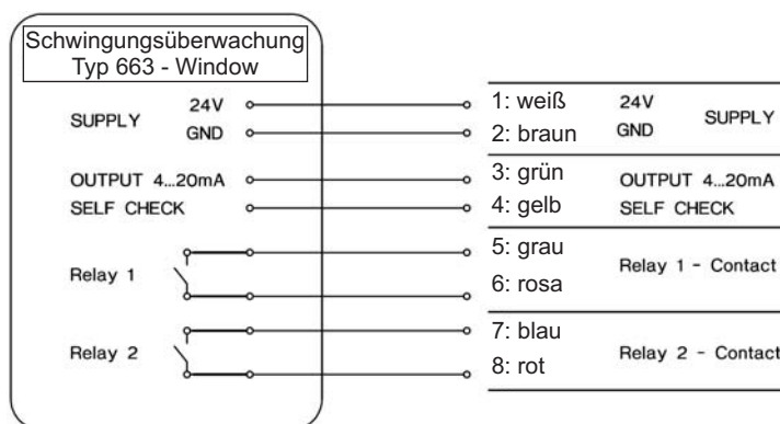
Abb. 8: Anschlussplan Typ 663 - Window
