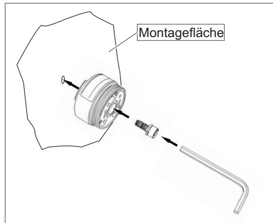
Abb. 12: Befestigung an der Montagefläche
