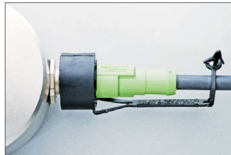
Abb. 15: Montierter Sicherungsclip
