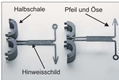
Abb. 14: Sicherungsclip
